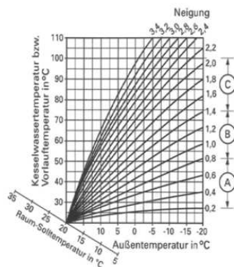
Einstellbare Heizkennlinien
