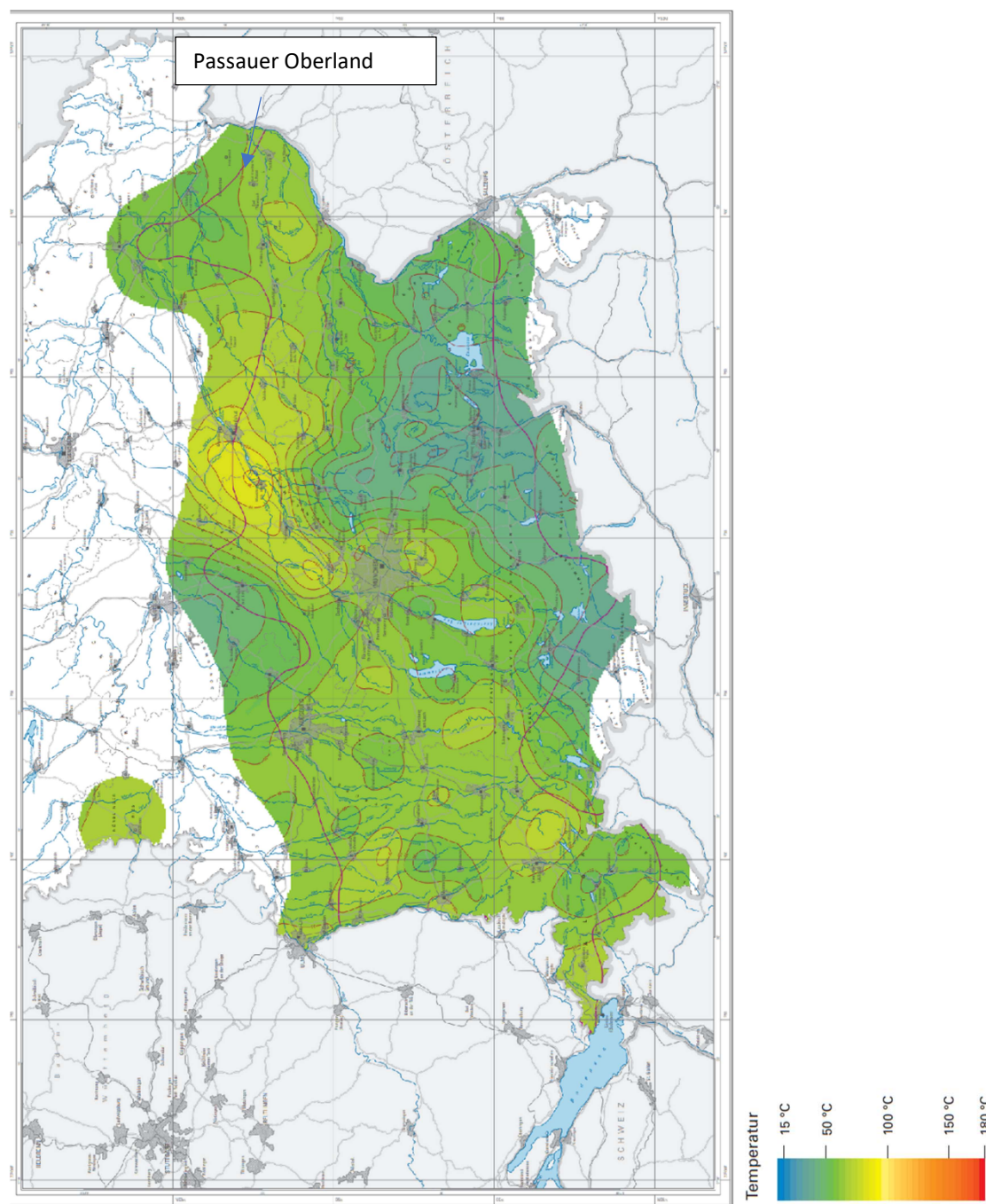
Abbildung 26: Geothermie Atlas
